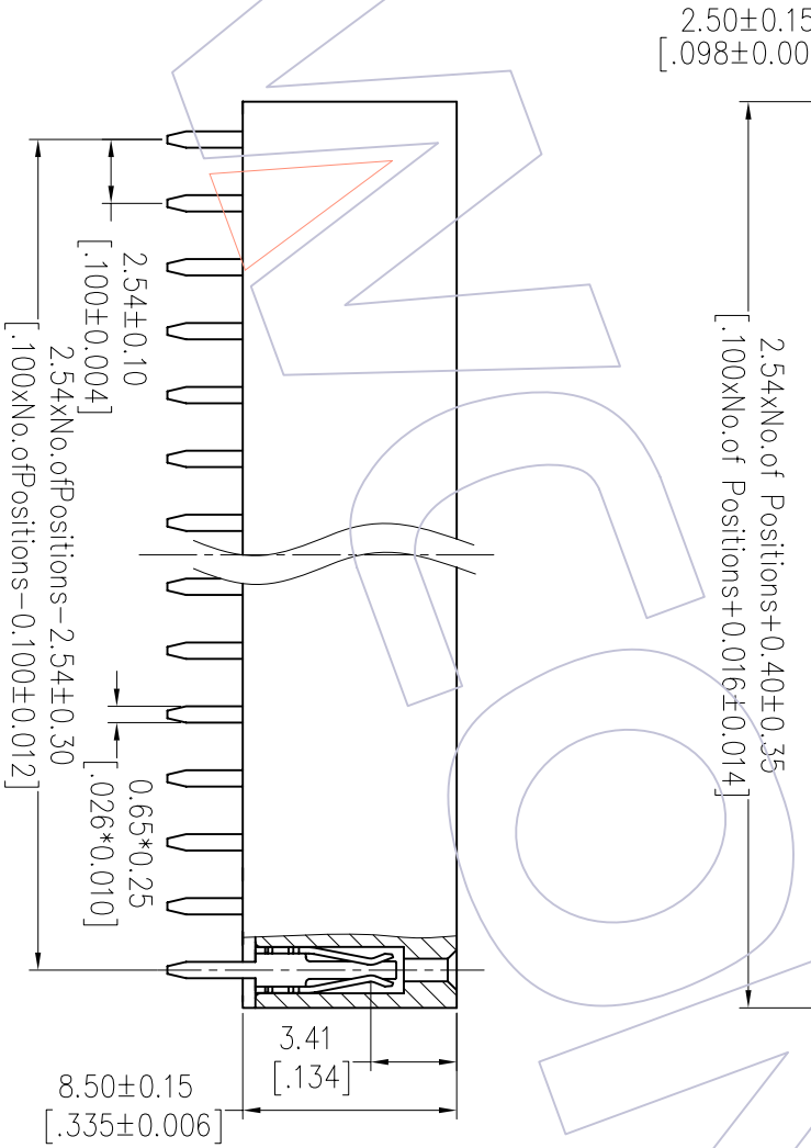
SECTION A-A
